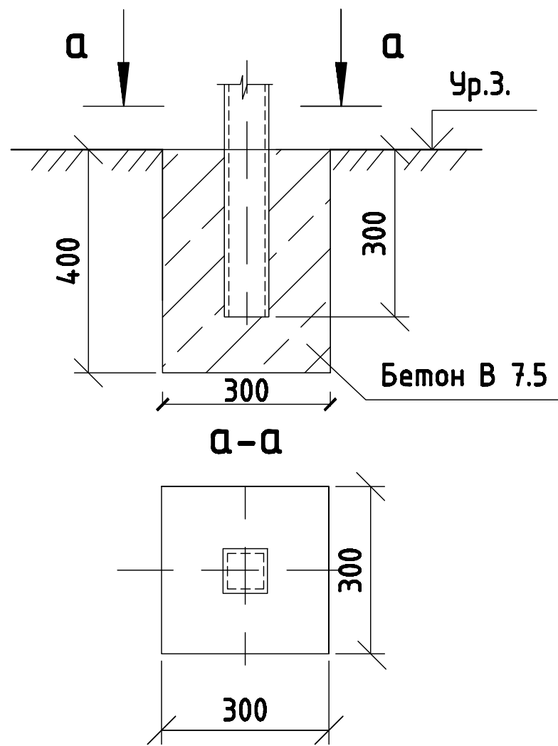
Фундамент под опоры скамеек и урн
